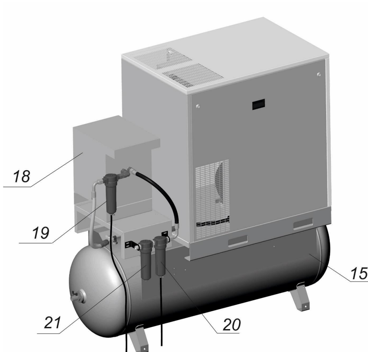
Рисунок 4 – Общий вид компрессорной установки BK20T-16-500Д2
