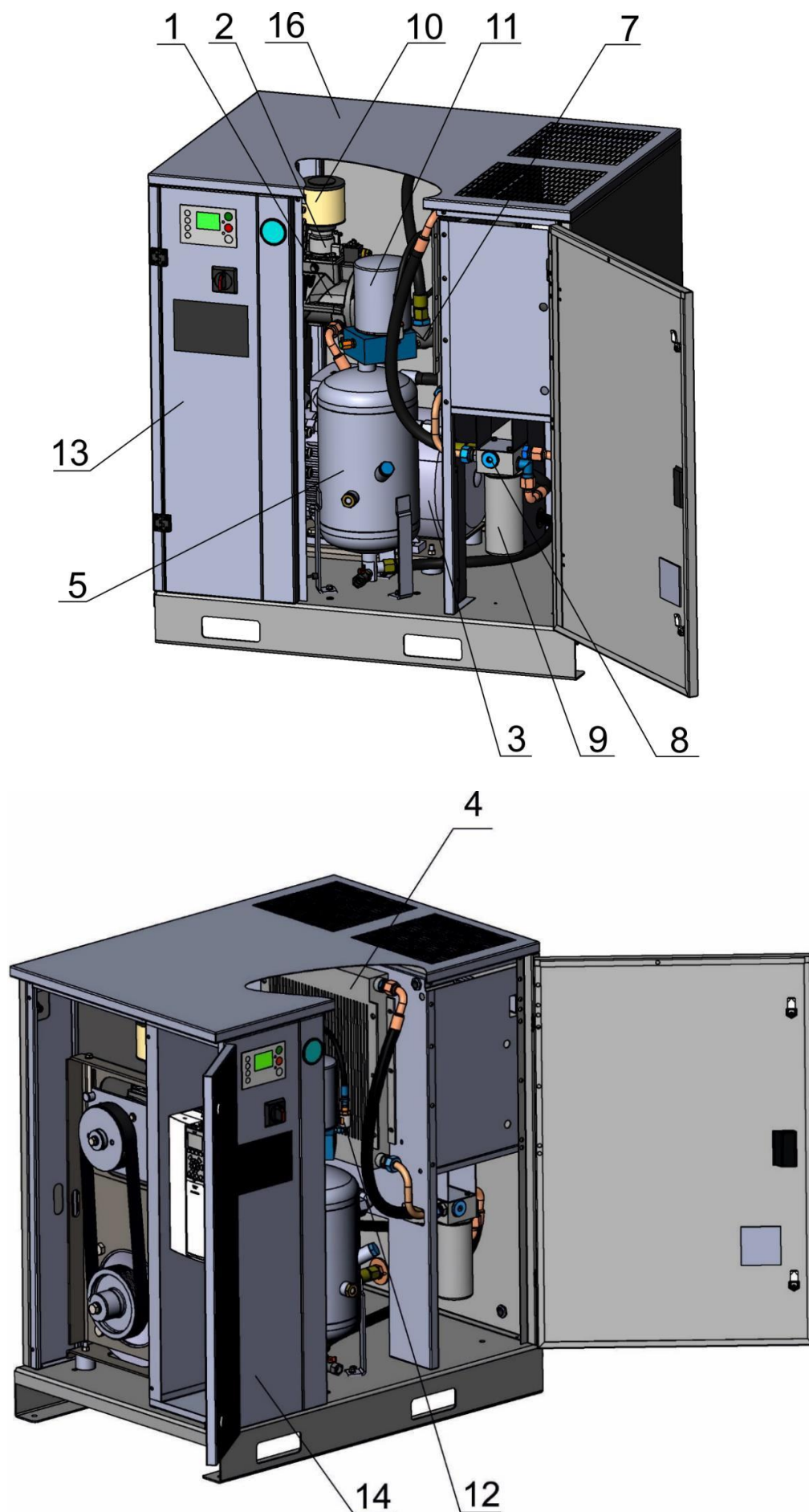
Рисунок 1.а – Общий вид компрессорной установки BK20T-8(10,16)
