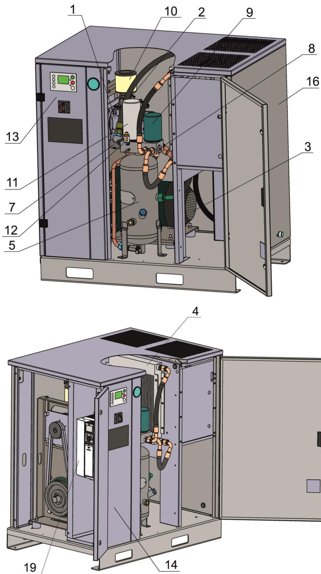
Рисунок 1.6 – Общий вид компрессорной установки BK20T-15
