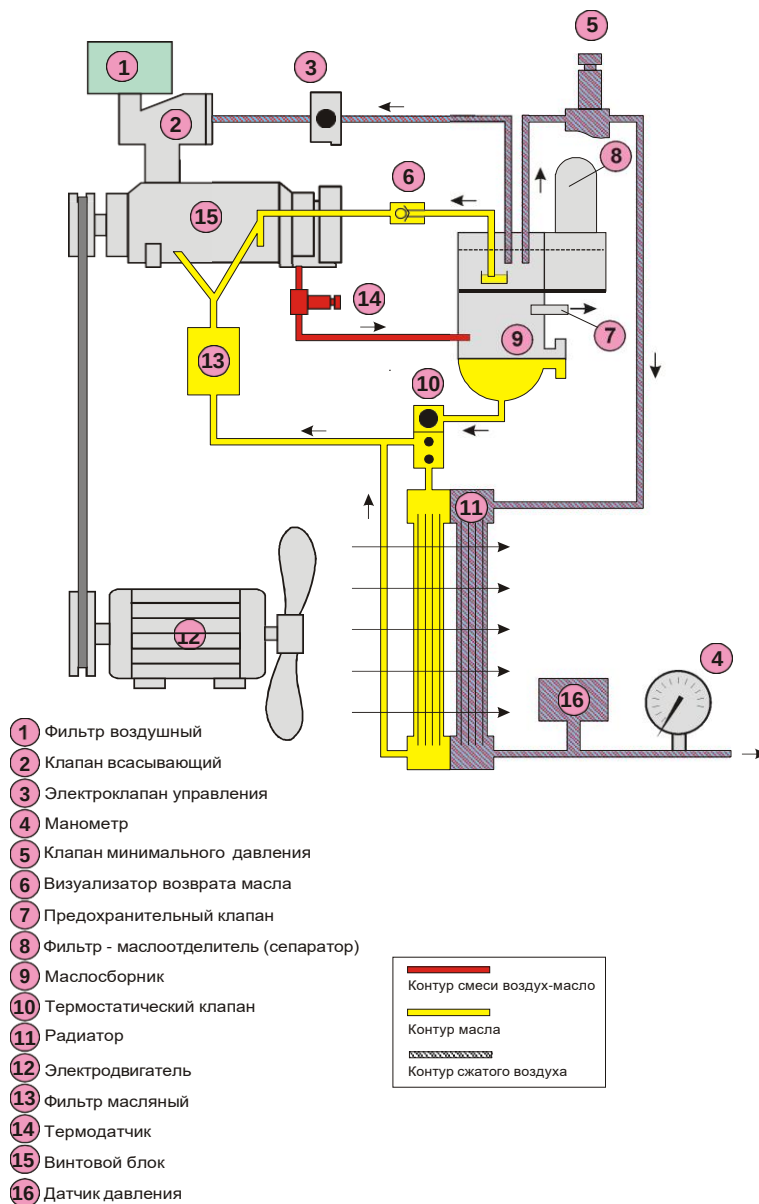
Рисунок 4 – Схема функциональная принципиальная компрессорных установок BK5E, BK7E, BK10E
