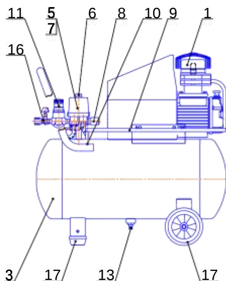
Рисунок 5 - Общий вид компрессора СБ4/С-24.J1047В
