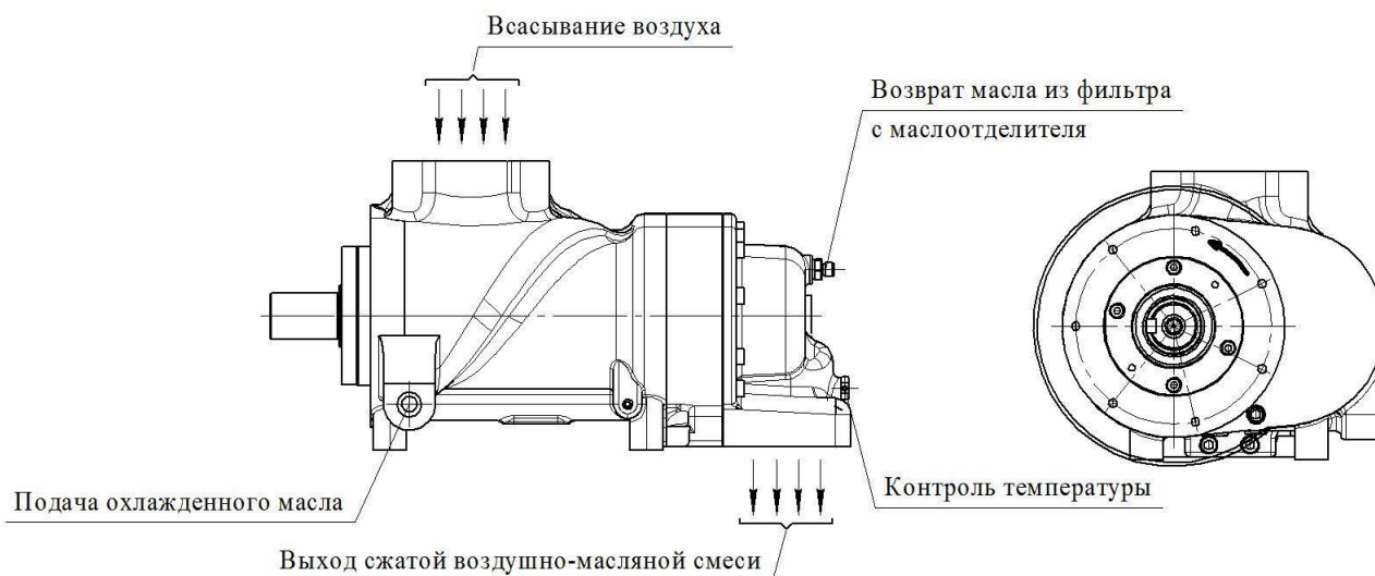
Общий вид блока винтового SCA14DR
